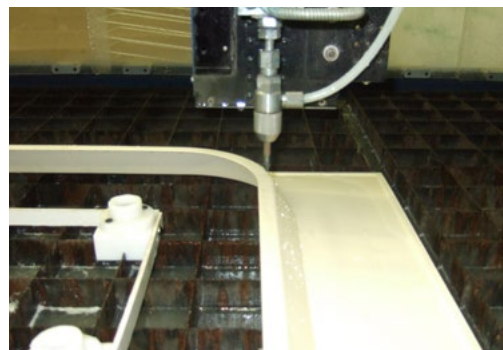
Waterjet
